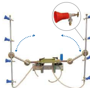
Barra múltiple 8 jets mariposa
